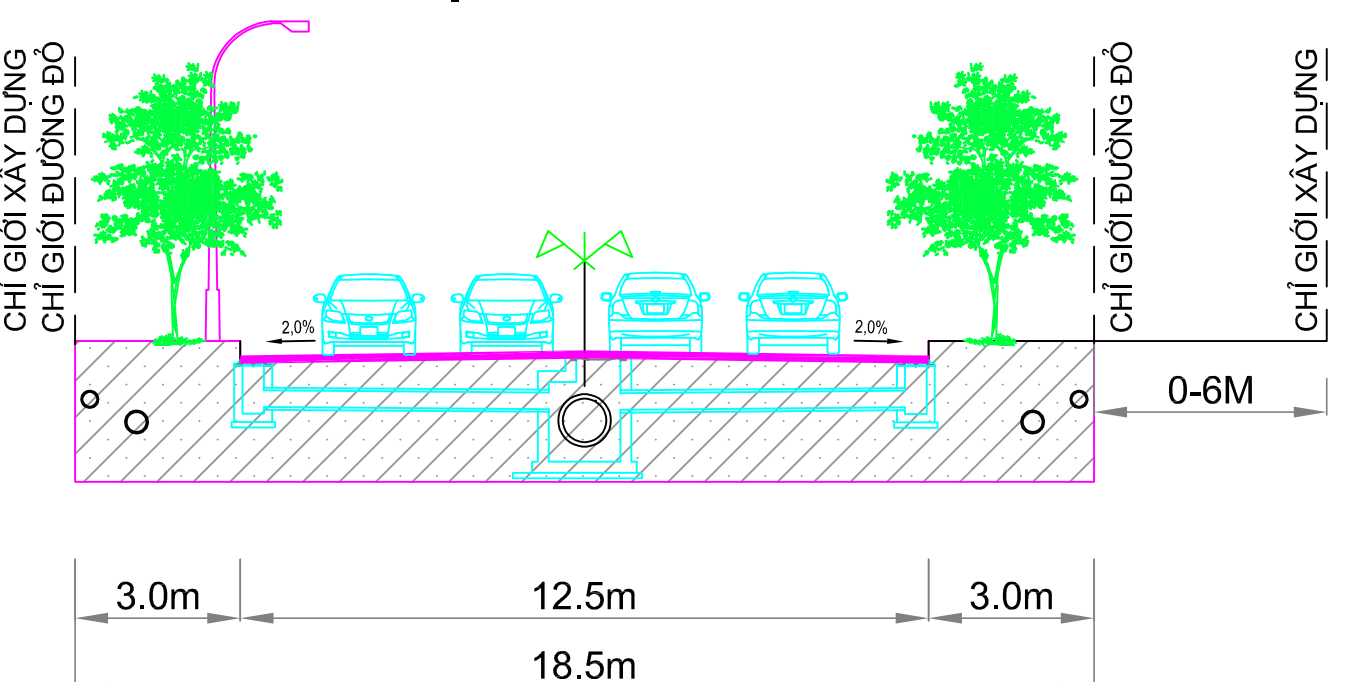
MẶT CẮT 1 - 1
