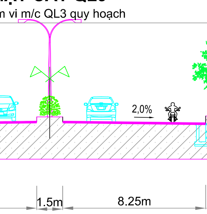
MẶT CẮT QL3
