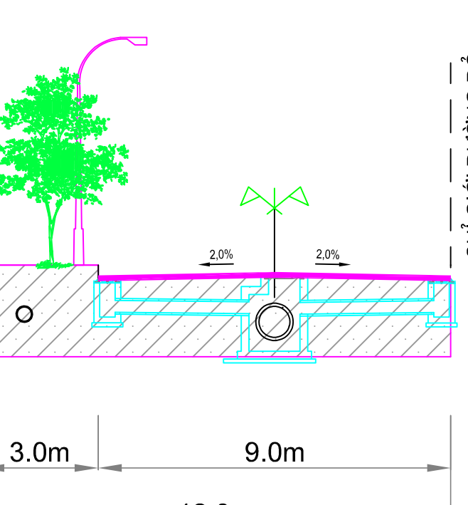
MẶT CẮT QL3
